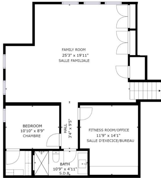
SURFACE INTÉRIEURE BRUTE/GROSS INTERNAL AREA (P.C/S.F.) (SOUS-SOL/BASEMENT - 923) (ÉTAGE/ FLOOR 1 - 1520)(ÉTAGE/FLOOR 2 - 987) TOTAL = 3431
