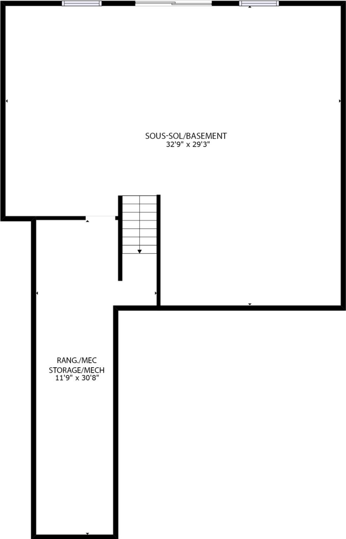
23 MORGAN, SENNEVILLE SURFACE INTÉRIEURE BRUTE/GROSS INTERNAL AREA (P.C/S.F.) (SOUS-SOL/BASEMENT - 1101) (REZ-DE-CHAUSSÉE/GROUND FLOOR - 1165) (ÉTAGE/FLOOR 2 - 1591) TOTAL = 3858
